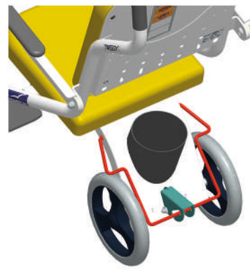
REF. 60145-01 PORTABOTELLAS ( Ø MAXI 155 )
